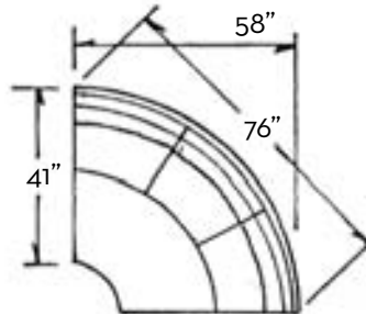
510-76W Wedge Section
