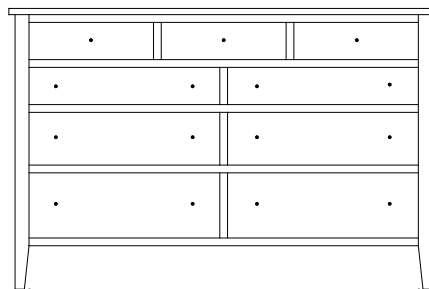
CS-1658 Dresser 69¼"w 45¼"h 21½"d w/9 drawers
