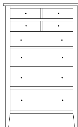
CS-1651 Hi-Boy 37¼"w 60¼"h 21½"d w/8 drawers
