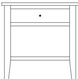
CS-1643 Night Stand 28"w 28"h 17½"d w/1 drawer
