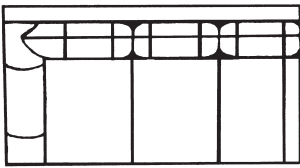
3570-1L LEFT ARM SOFA H36 W80 D38 INSIDE: H16 W70 D22 SEAT H: 20 ARM H: 22
