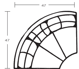
3579 WEDGE H36 W74 D41 INSIDE: H16 W56 D22 SEAT H: 20
